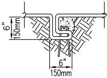
CHECK SLOT
