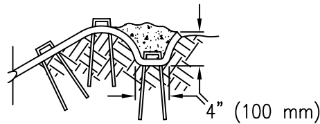
LONGITUDINAL ANCHOR TRENCH
