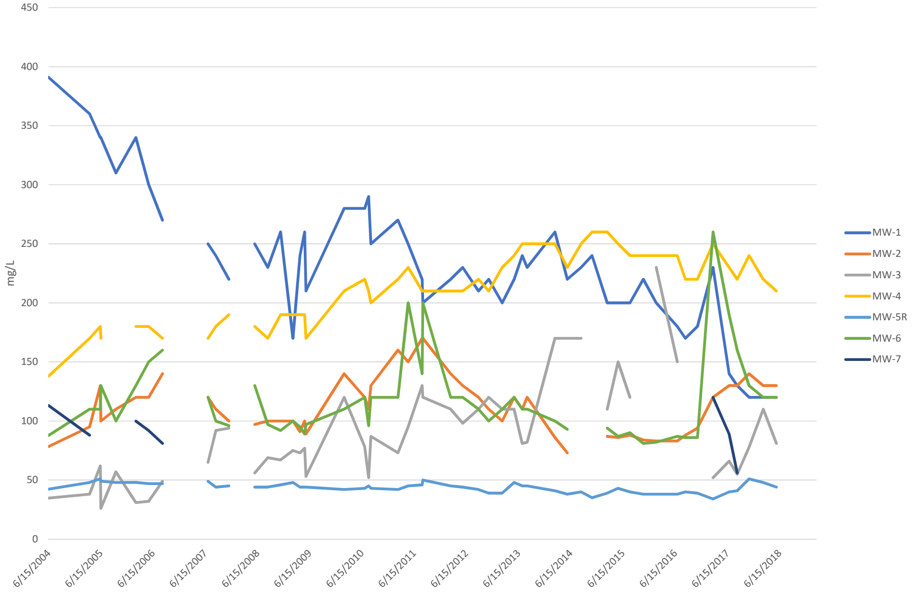
Chart 5 CI Trends 2004-19
