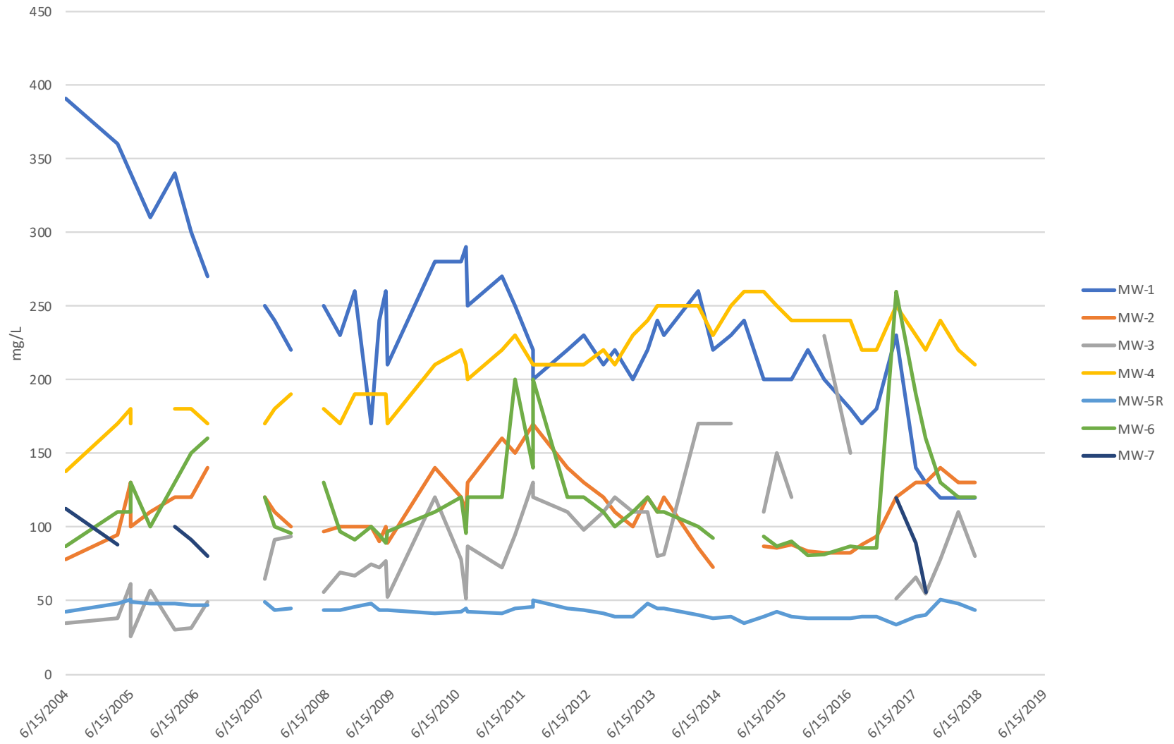
Chart 5 CI Trends 2004-19
